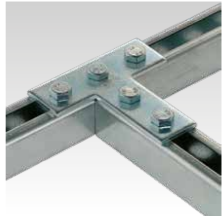
T-Verbindungsplatte
